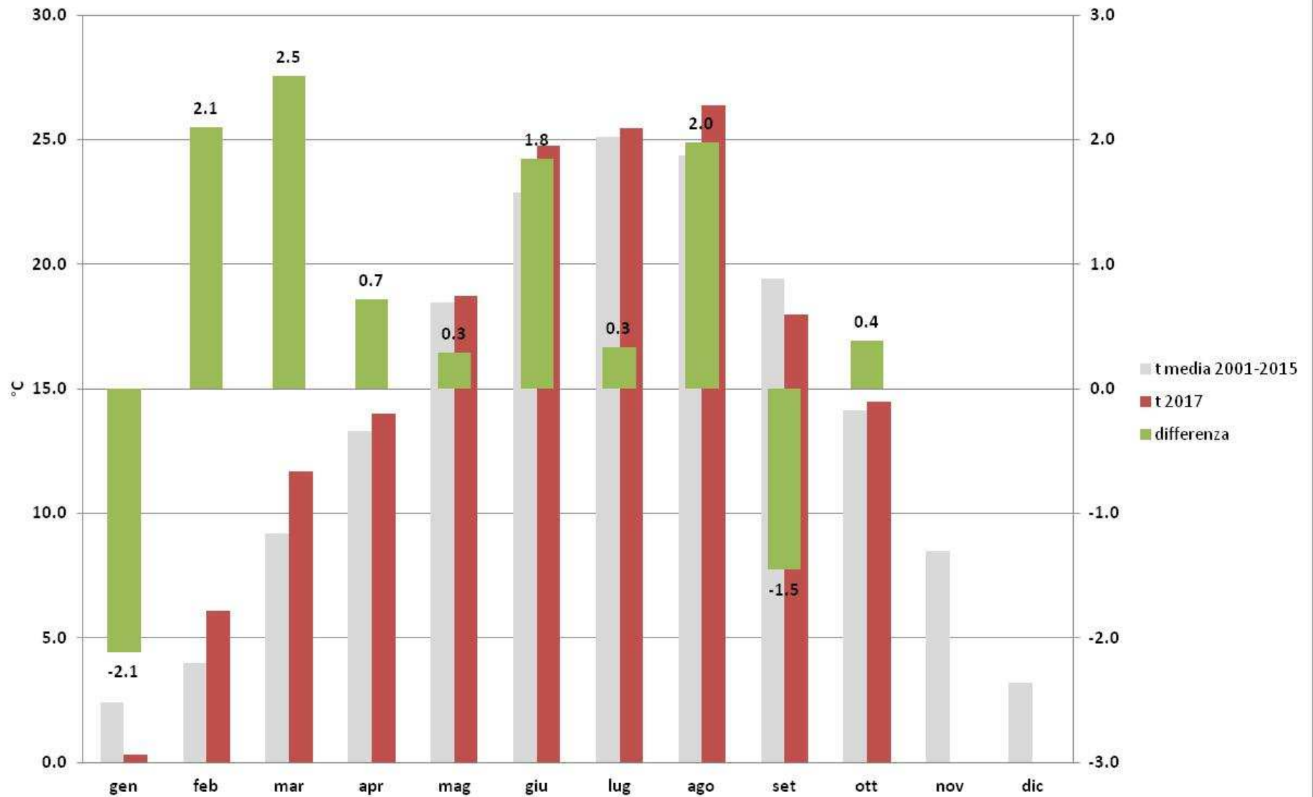
S.Pancrazio: tmed mensile 2017 e media 2001-2015
